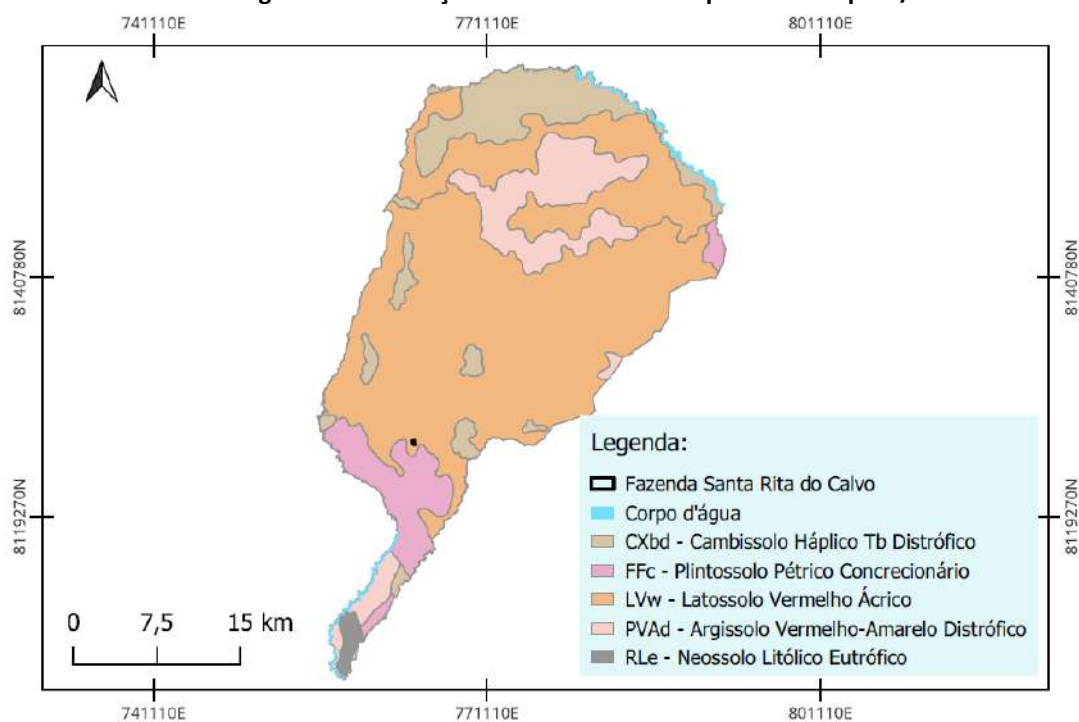
Figura 2. Distribuição dos solos no Município de Vianópolis/GO
