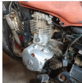
MOTOR COMPARTIMENTO
